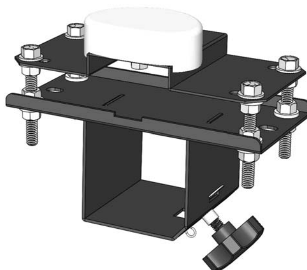
V2P-TAGLESS Pallet Arm P/N: V2-ARM-M
